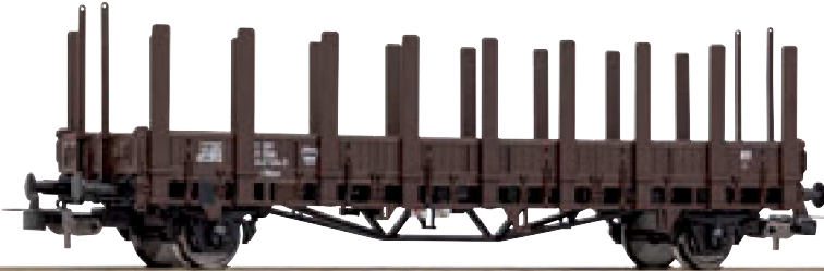
24521 Rungenwagenx „Ulm“ ÖBB Ep. IV
